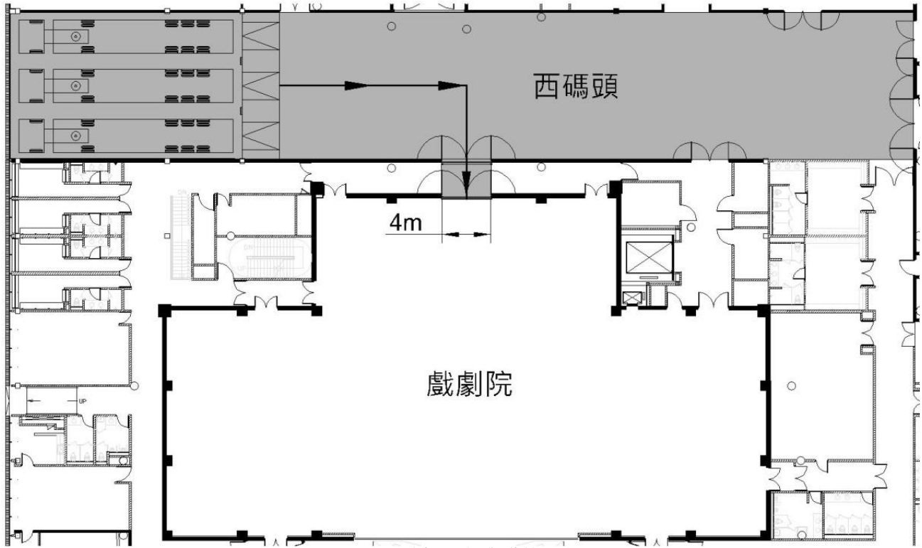
圖例 4.3 卸貨動線
