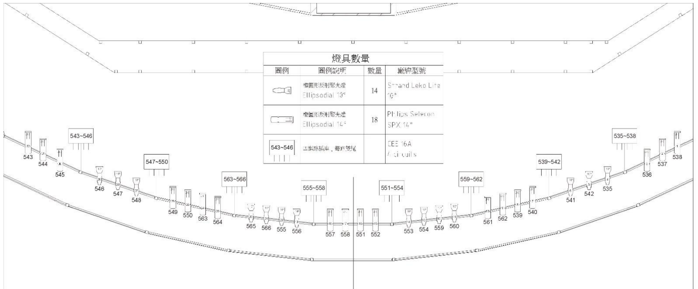
圖例 2.1 外區燈具配置圖
