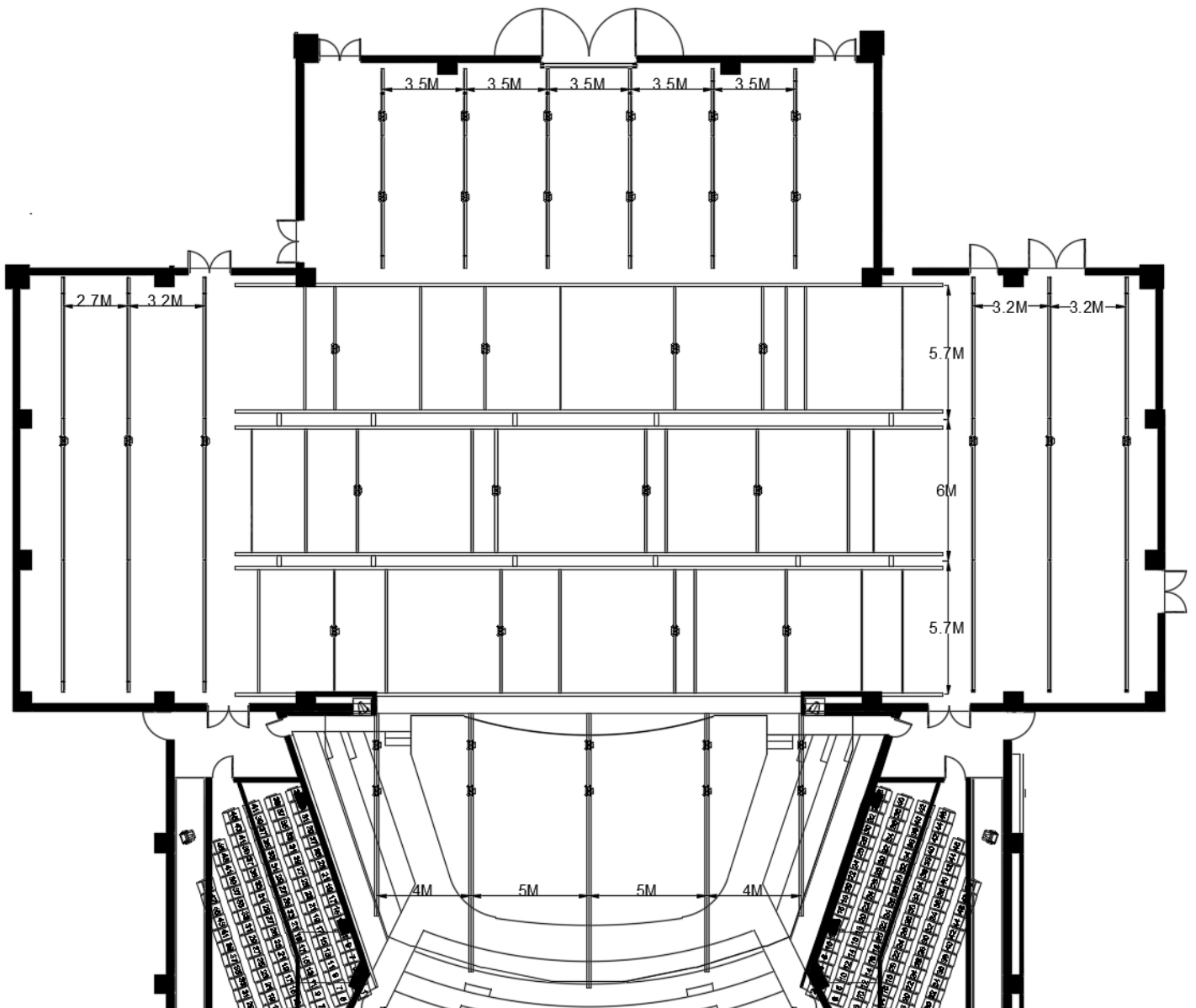
圖例 1.6 鍊條馬達位置
