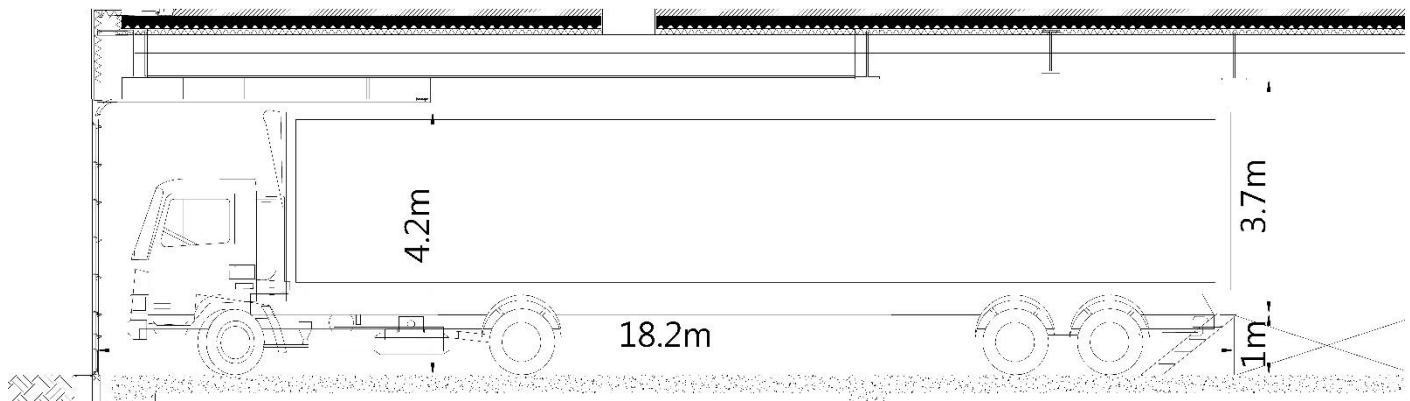
例 4.2 西碼頭卸貨口剖面圖
