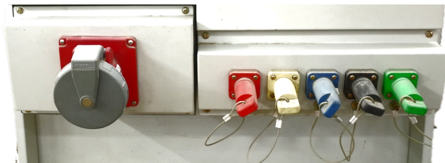
圖例 2.4 外接電源 Camlock、CEE125 圖示
