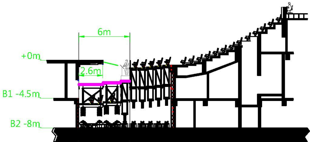
圖例 1.2.1.2-樂池升降平台剖面圖
