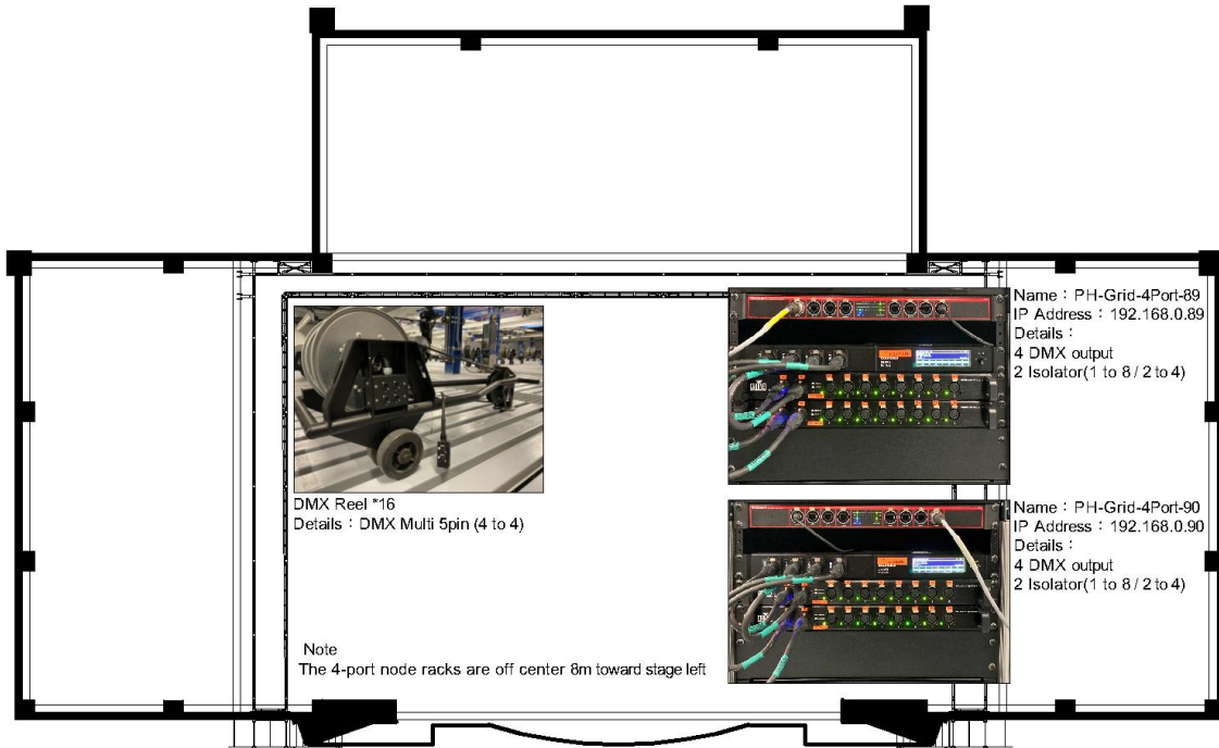
頂棚區 Node 位置圖
