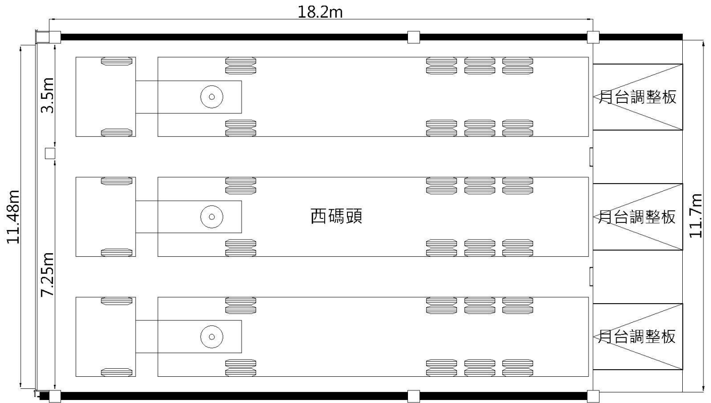
圖例 4.1 西碼頭卸貨口平面圖
