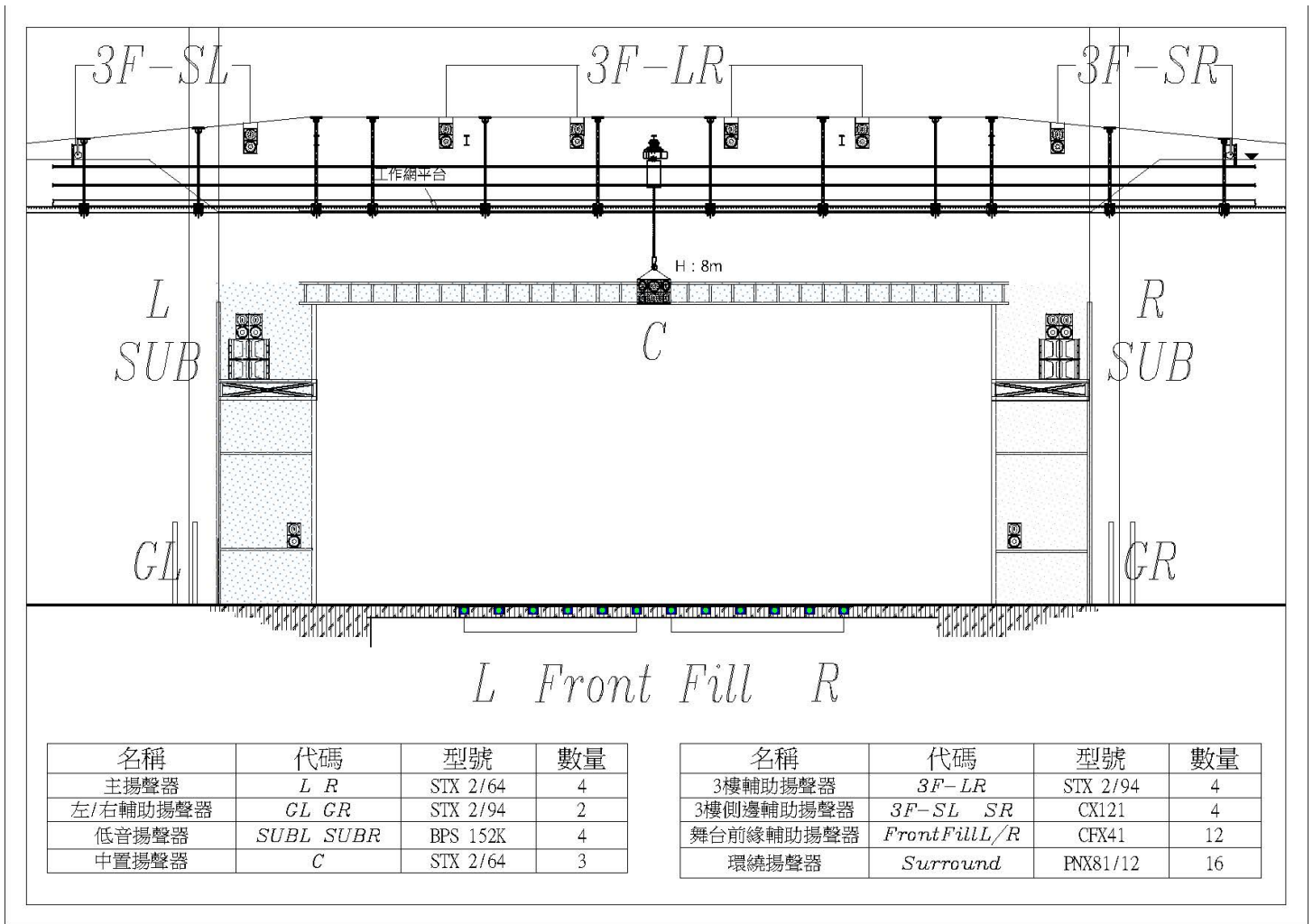
圖例 3.1 揚聲器配置立面圖
