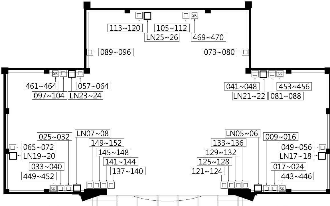
圖例 2.3.1 舞台區迴路配置
