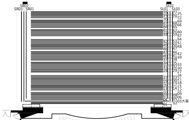
圖例 1.5.1-吊桿平面圖
