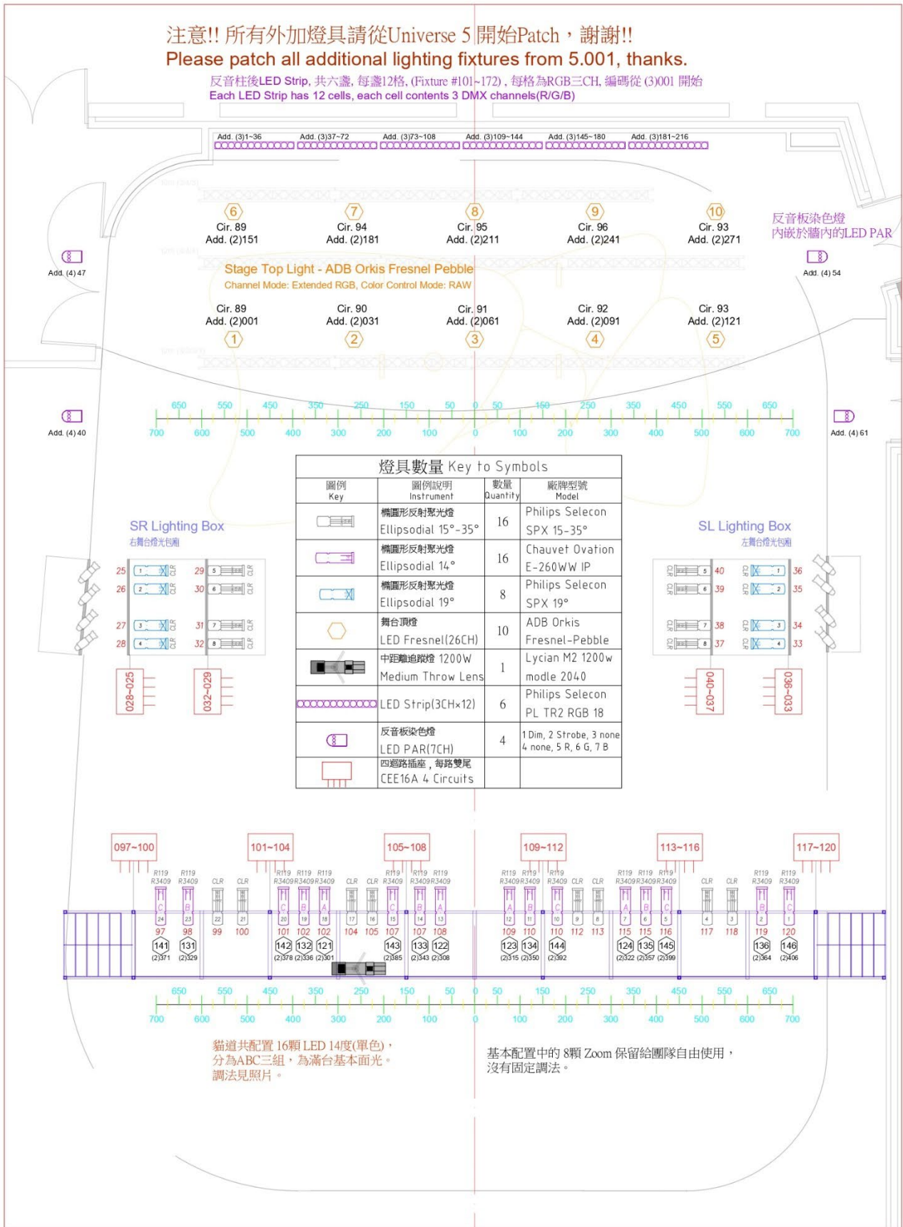
衛武營表演廳 Recital Hall 燈具迴路配置圖
