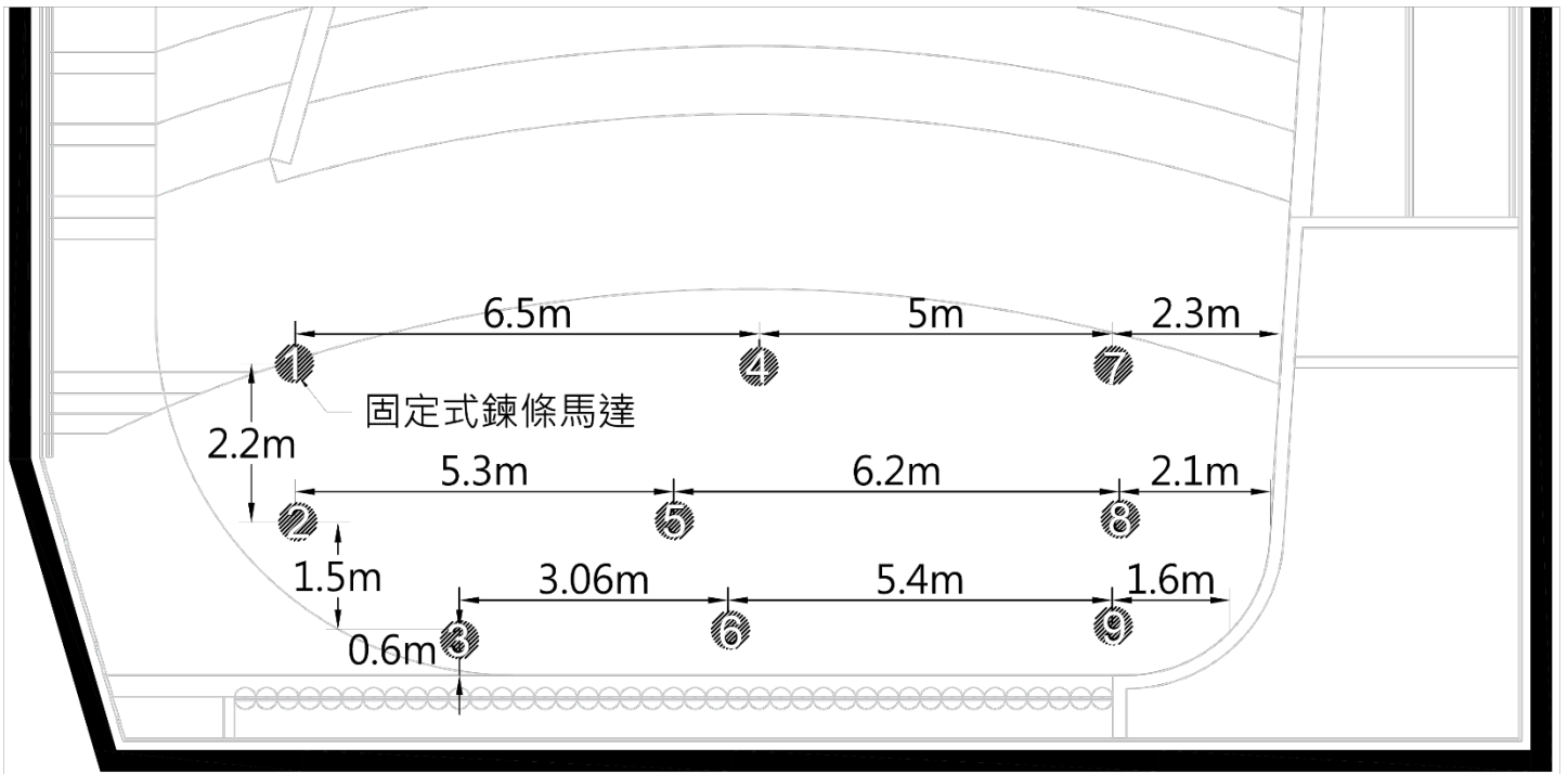
圖例 1.4 鍊條吊車位置圖
