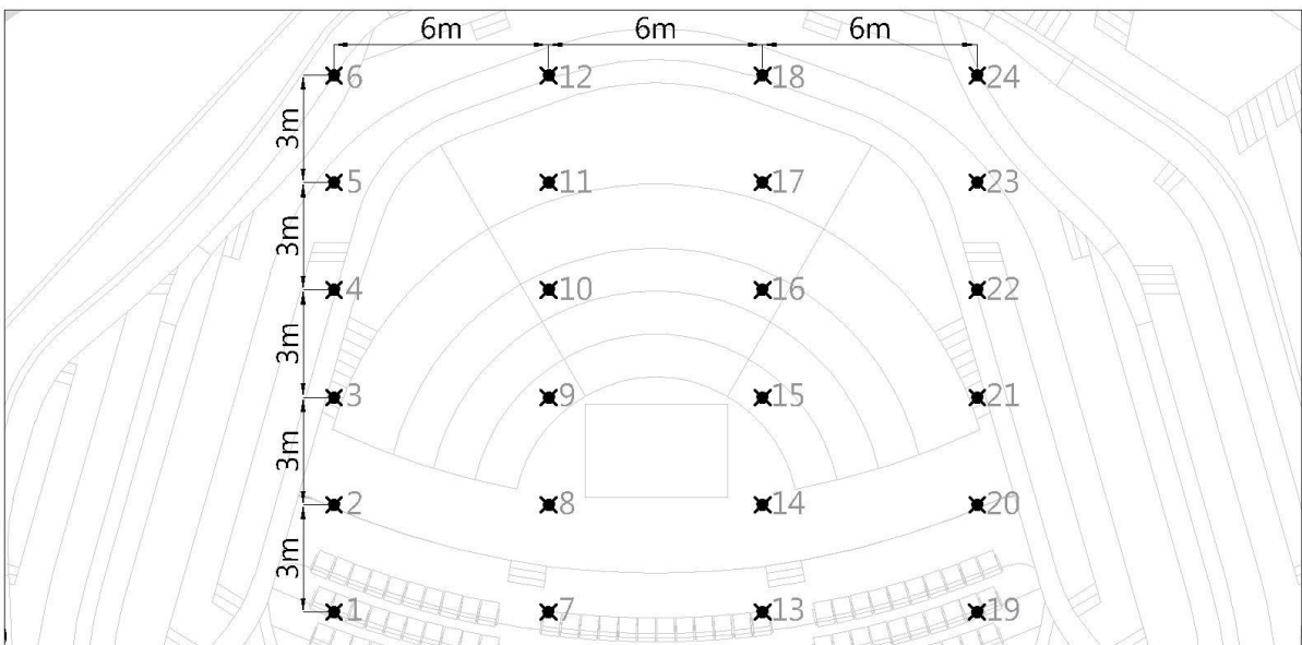
圖例 1.2 鍊條馬達位置圖
