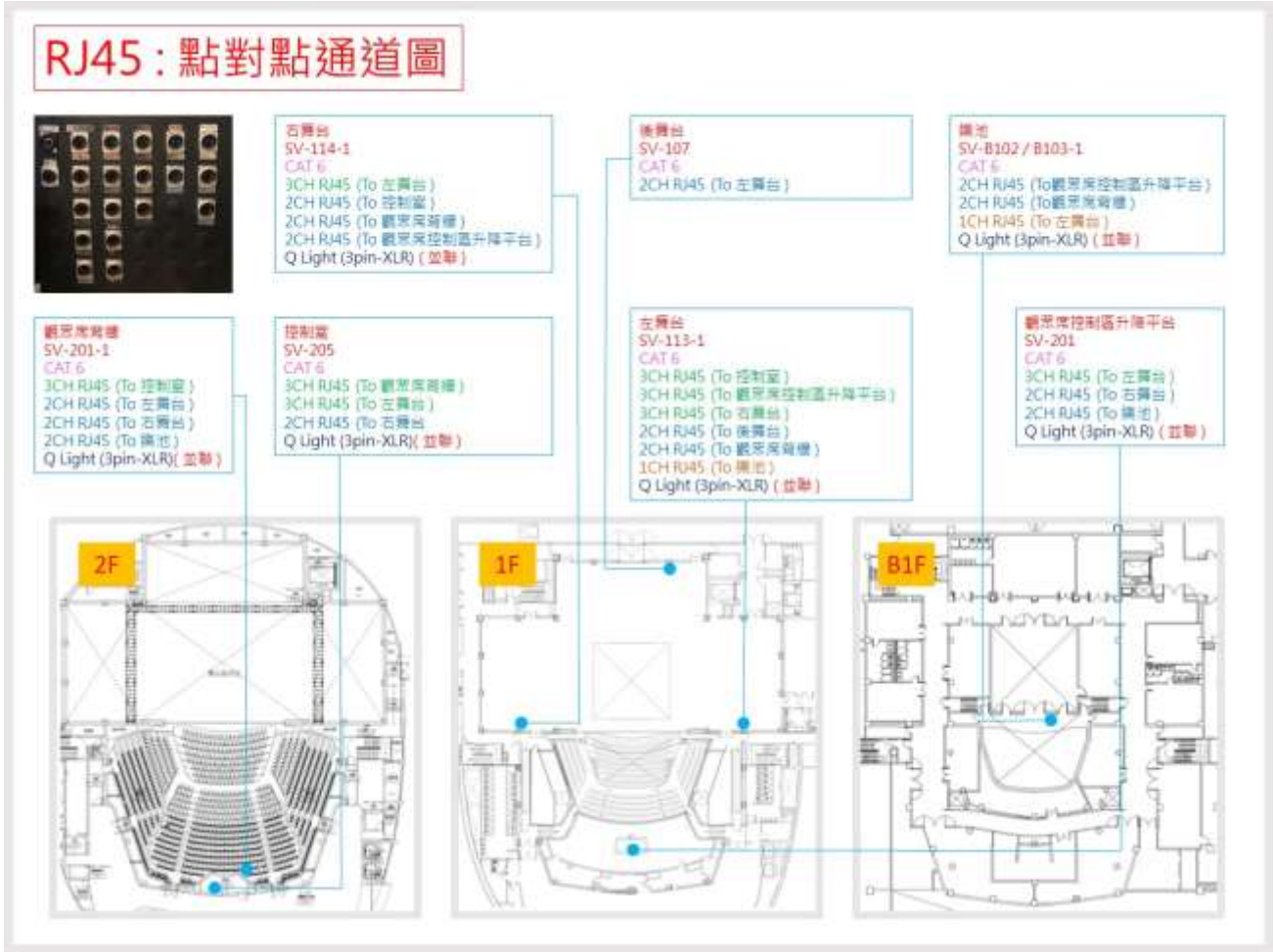
圖例 4-1.8 RJ45 信號通道圖示
