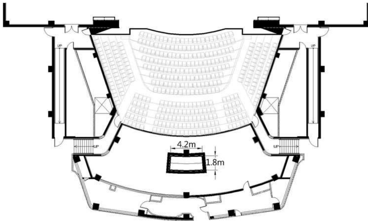
圖例 2.2.4-觀眾席控制區位置圖
