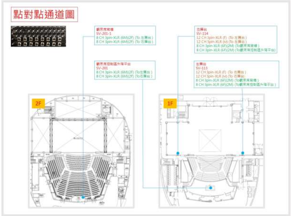
圖例 4-1.7 信號通道圖示
