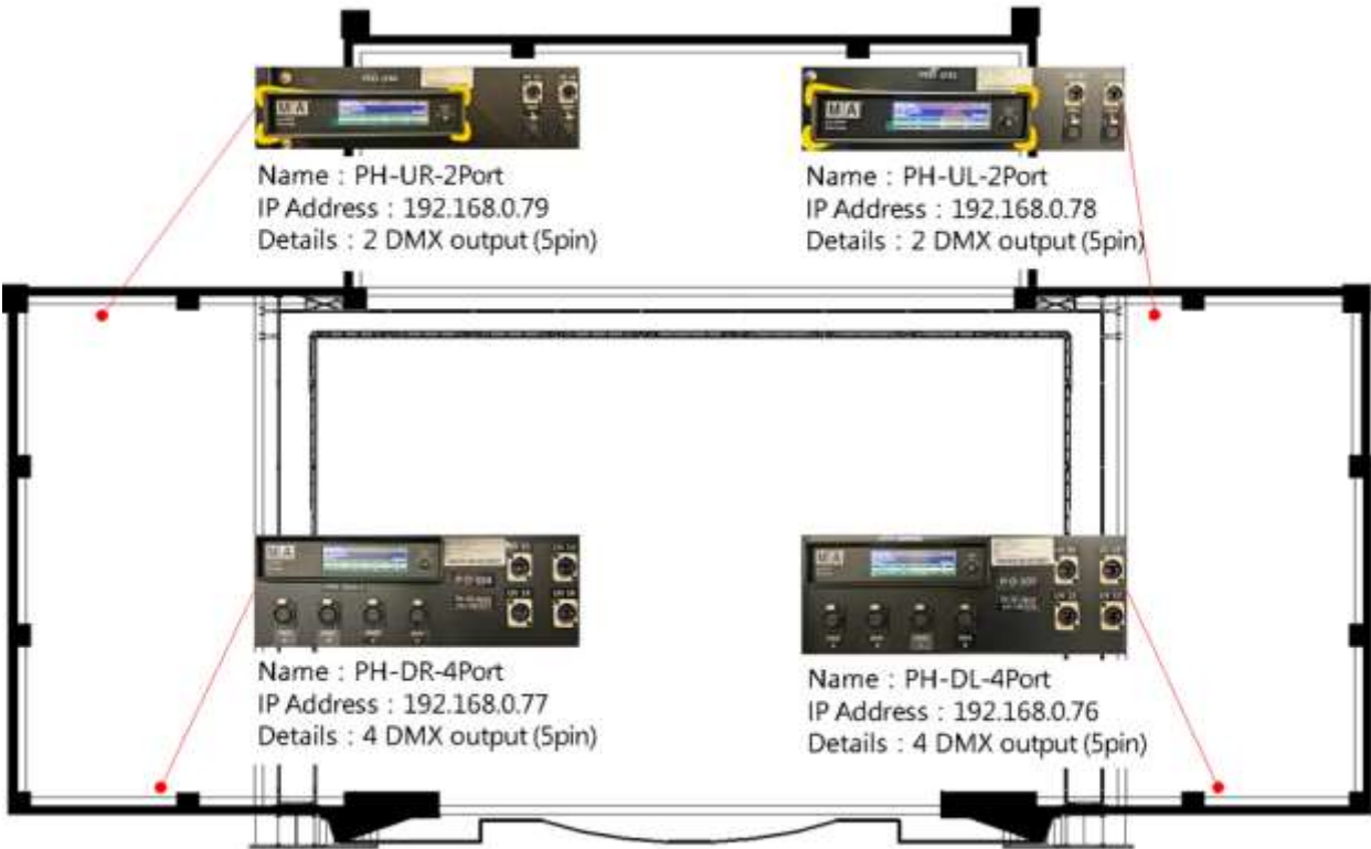
圖例 3.3.2- 舞台區 Node 位置圖
