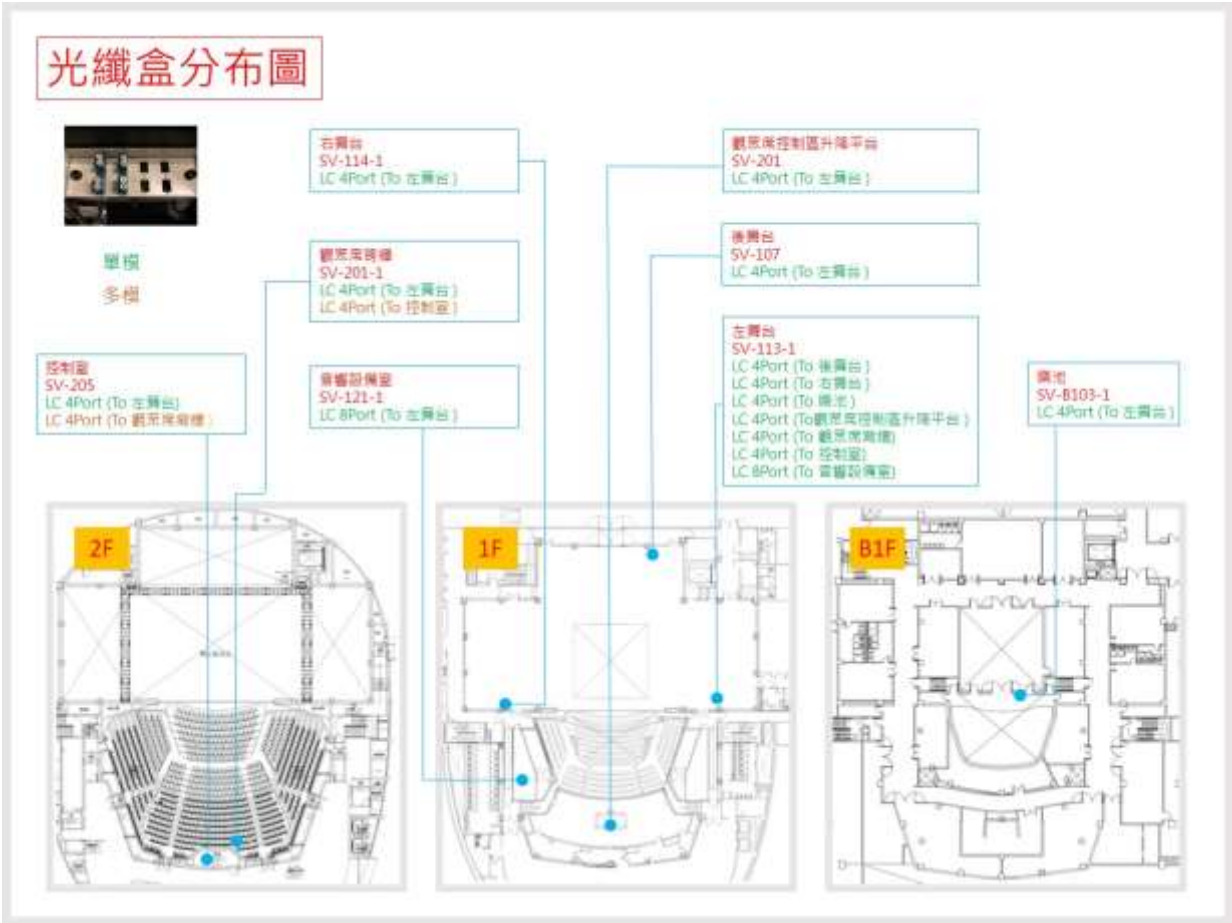
圖例 4-1.6 光纖通道圖示
