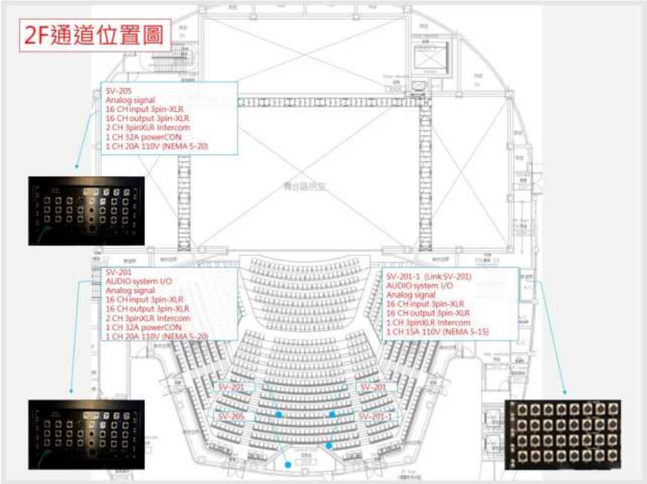
圖例 4-1.4 音響 2F 通道圖示
