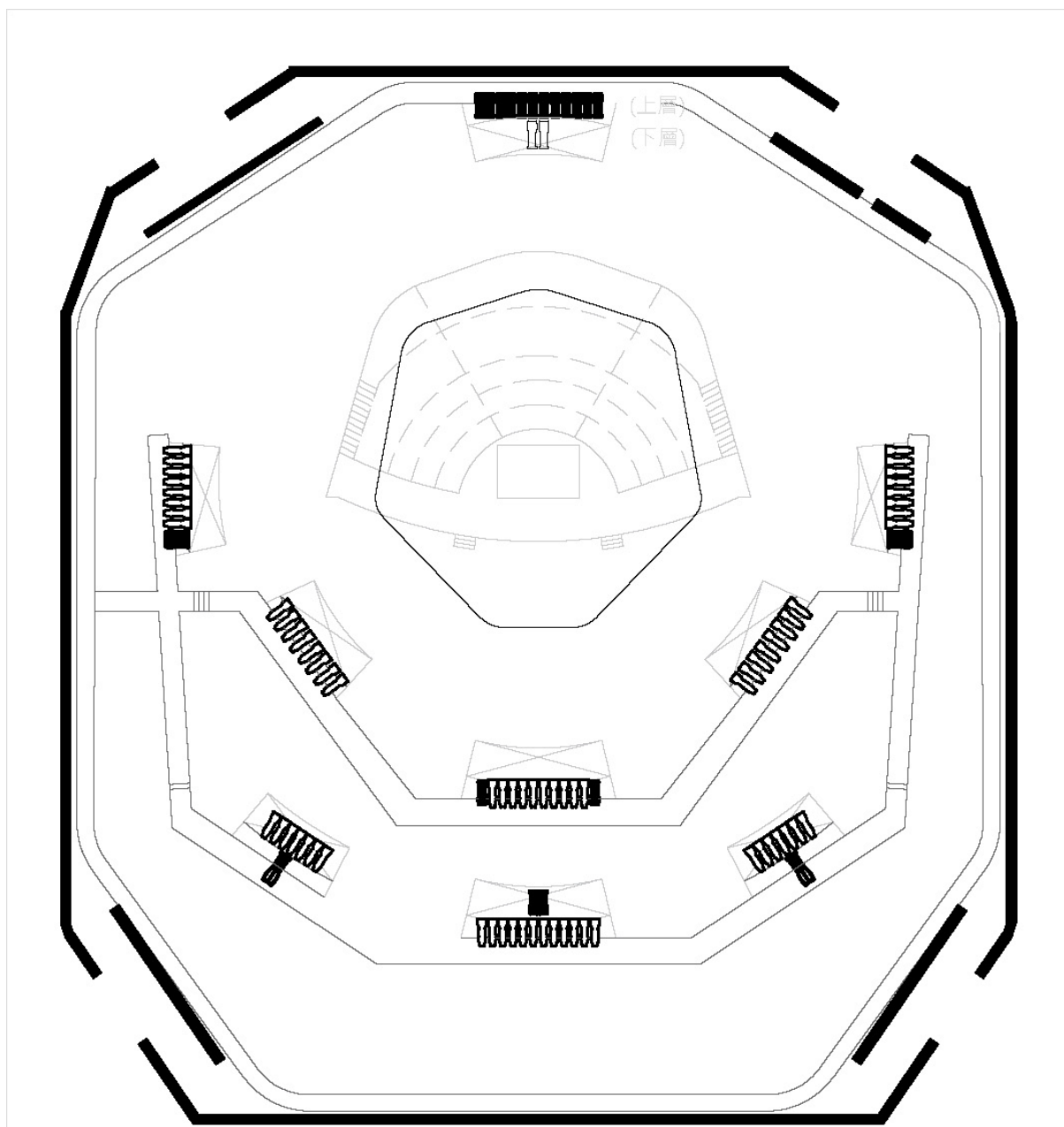
圖例 2.2 外區燈具配置圖
