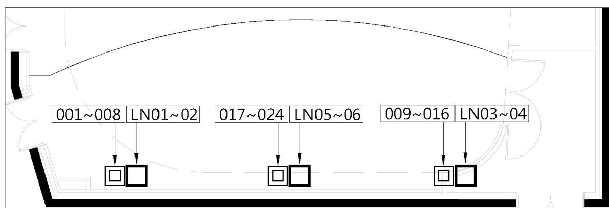
圖例 2.3.1 舞台區燈光迴路配置
