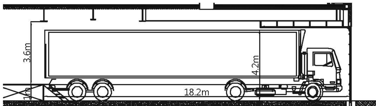
圖例 4.2 東碼頭卸貨口剖面圖
