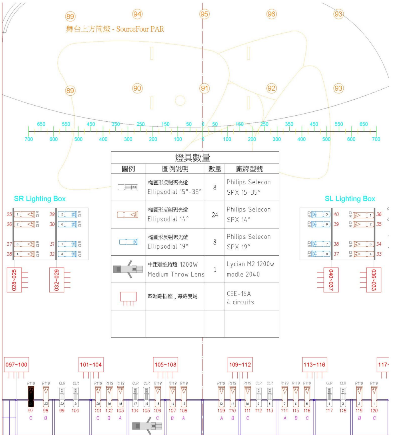
圖例 2.1 燈具配置圖
