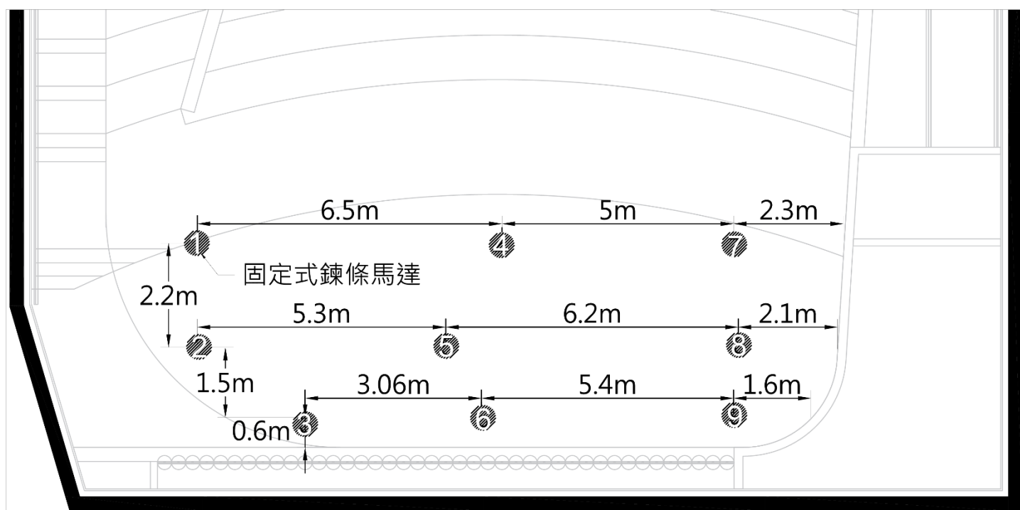
圖例 1.4 鍊條吊車位置圖
