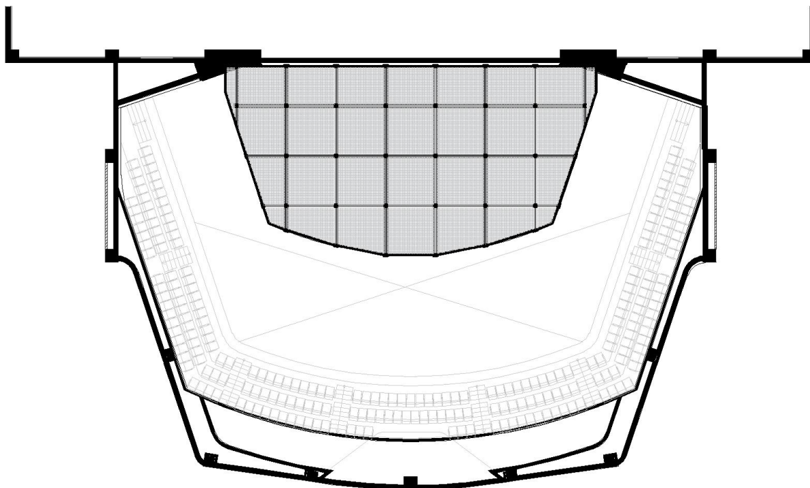
圖例 1.4-張力索棚架位置圖
