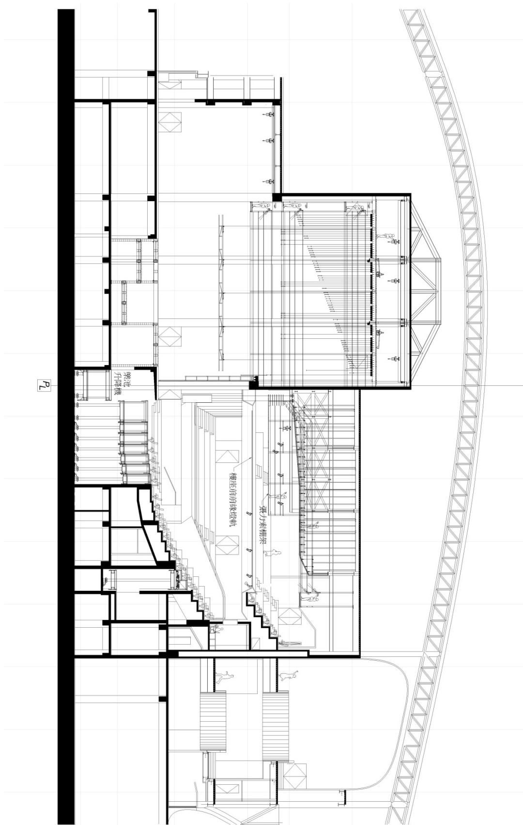
圖例 0.3-戲劇院剖面圖
