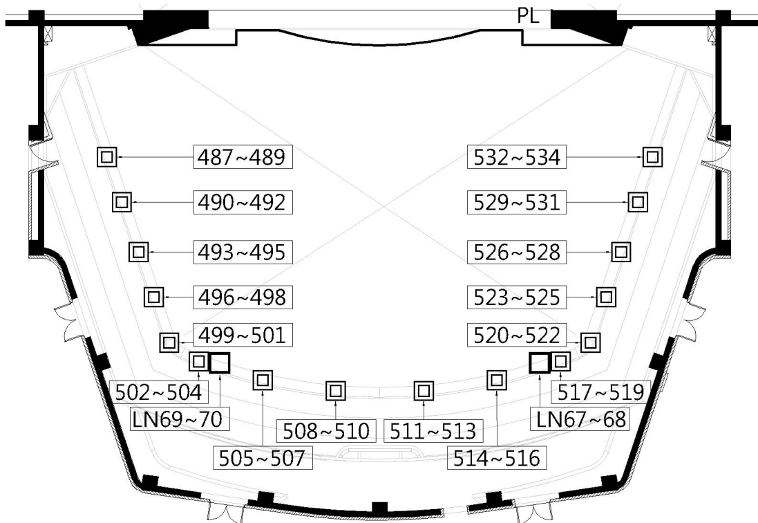
圖例 2.3.6 樓座前緣迴路配置
