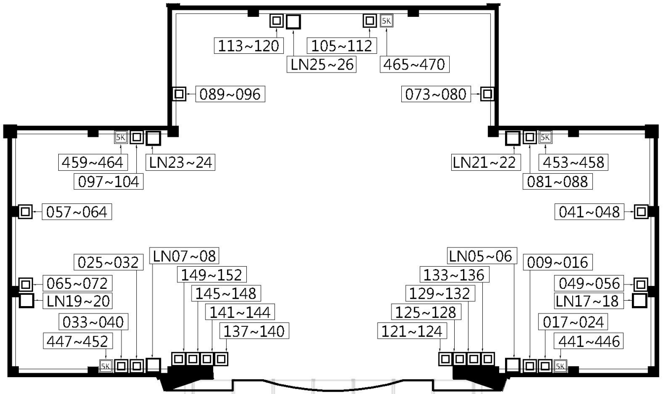
圖例 2.3.1 舞台區迴路配置
