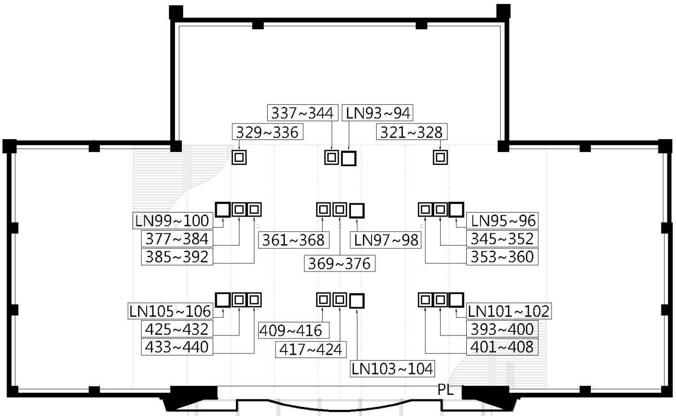
圖例 2.3.3 舞台頂棚區燈光迴路配置
