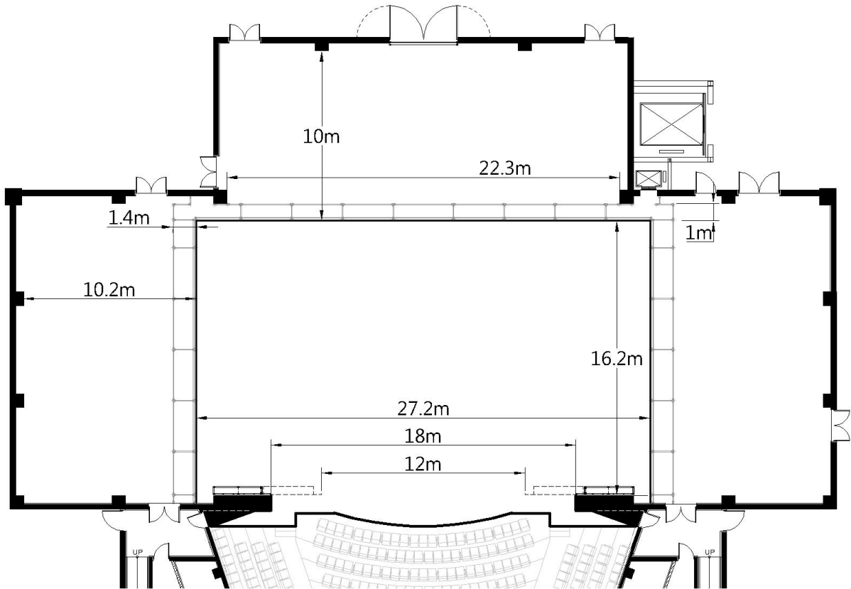
圖例 1.1-舞台平面圖
