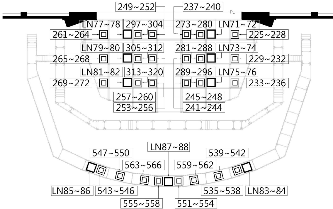
圖例 2.3.5 張力索棚架與貓道迴路配置
