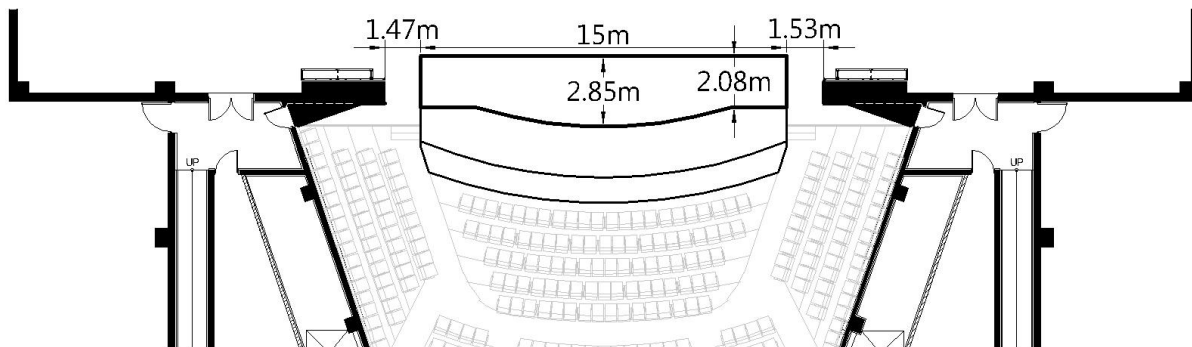
圖例 1.2.1.1-樂池升降平台位置圖
