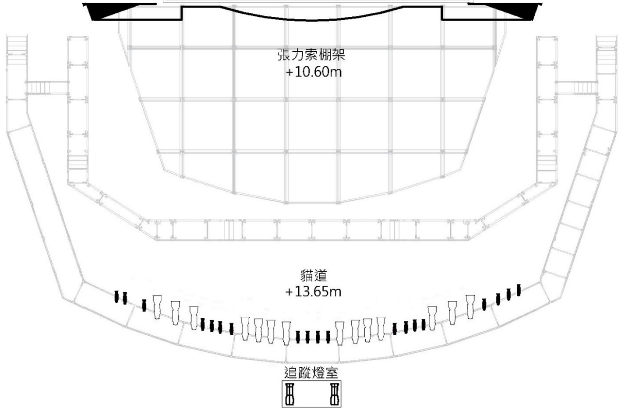
圖例 2.1 外區燈具配置圖
