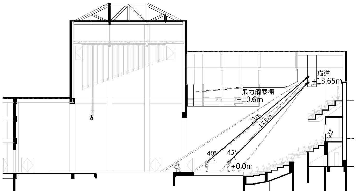
圖例 2.2-燈光剖面圖
